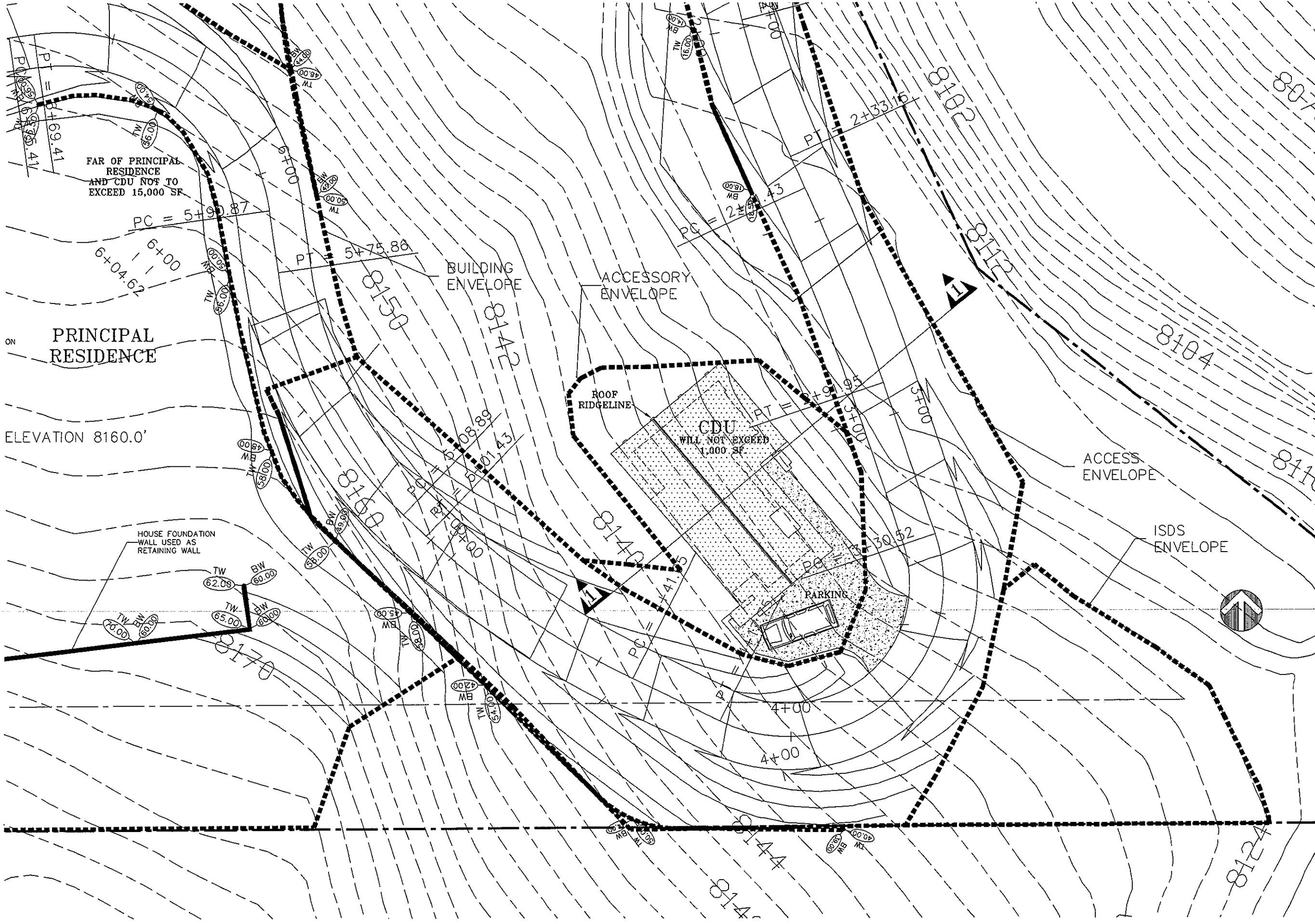
1 SITEPLAN SCALE: 1"=10'
